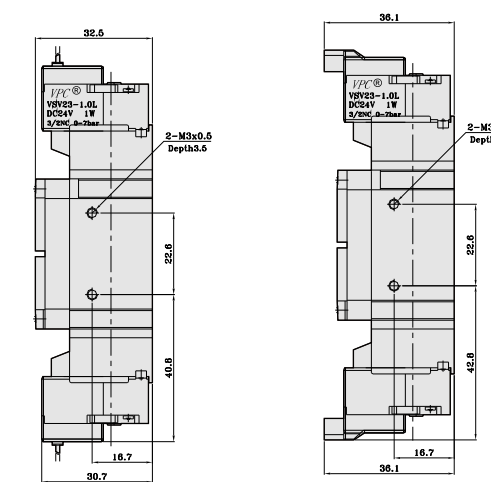
SY5220-G
