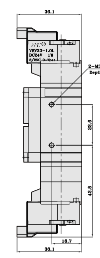
3 SY5420-M 5
