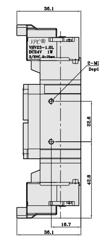
SY5220-M
